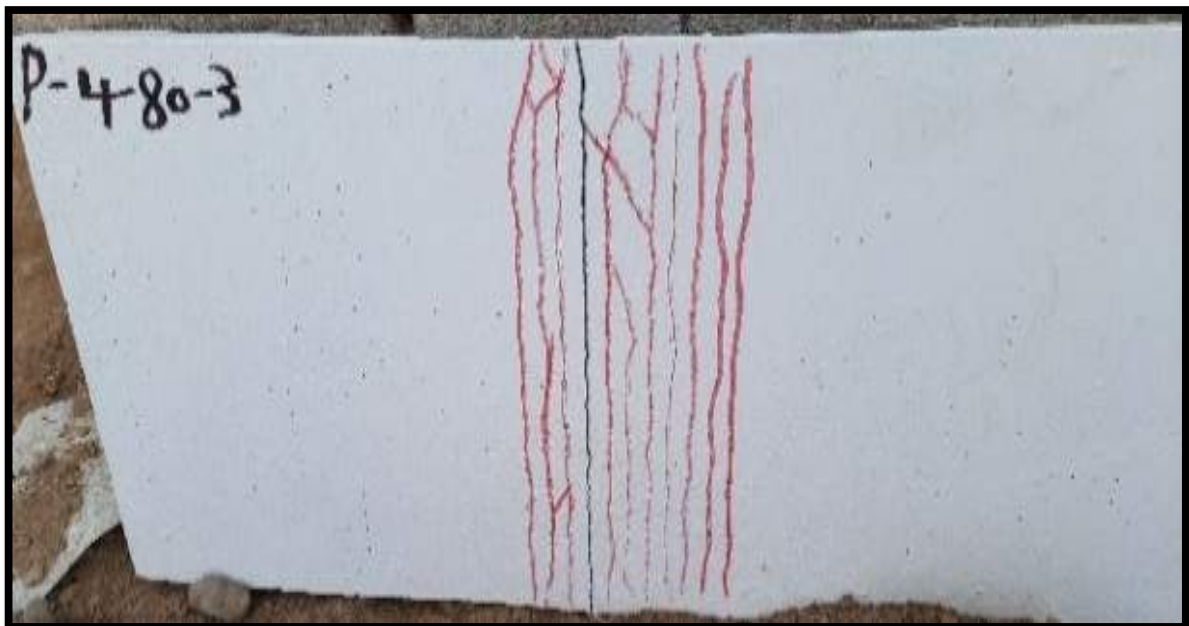
(d) Mode of failure for P-4-80-3 specimen.
